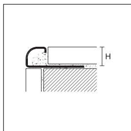
RIN/10 stainless steel AISI 304 - DIN 1.4301
