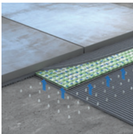
PWP30 - vapour vent
