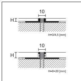
NTA/10 natural aluminium + EPDM grey polishable RAL 7046
