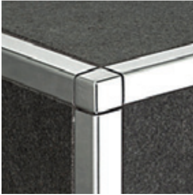
ZQIN/10/EI stainless steel AISI 304 - DIN 1.4301
