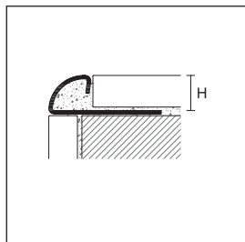
RI/10 stainless steel AISI 304 DIN 1.4301
