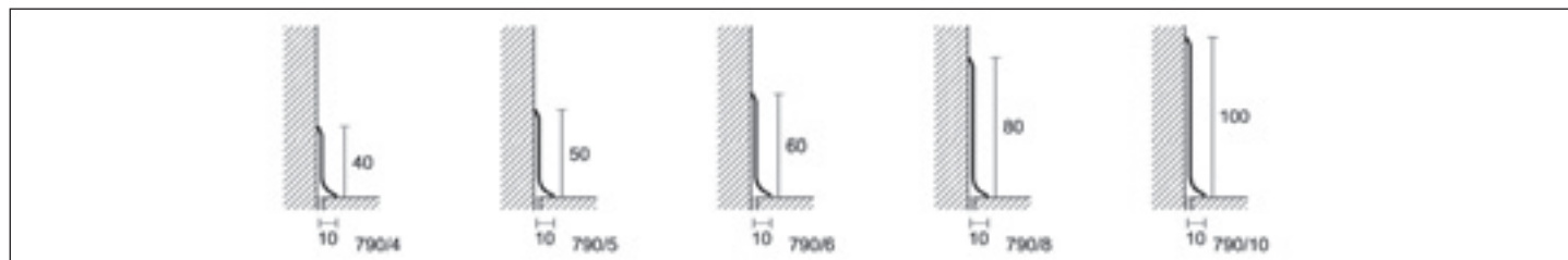
790/6 satin stainless steel AISI 304 DIN 1.4301
